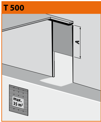
T 500 Verticaal railsysteem A= daghoogte + 560 mm
