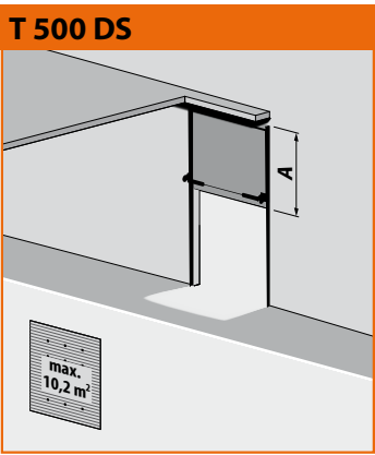
T 500 DS Verticaal railsysteem met laagliggende veeras A= daghoogte + 400 mm Breedte max. 3.200 mm Hoogte max. 3.200 mm
