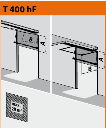
T 400 hF Verhoogd railsysteem met laagliggende veeras + stalen draagprofiel A= heffing + 200 mm, B= daghoogte – heffing + 600 mm Breedte max. 4.500 mm Heffing min. 1.450 mm
