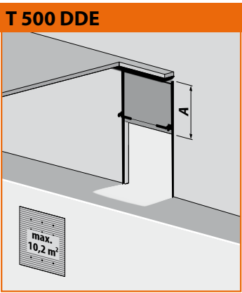
T 500 DDE Veerloze verhoogd railsysteem A= daghoogte + 400 mm Breedte max. 3.200 mm Hoogte max. 3.200 mm
