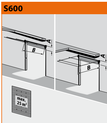
S600 Helix S600 Horizontaal railsysteem A= 600 mm B= daghoogte + 265 mm Breedte max. 5000 mm
